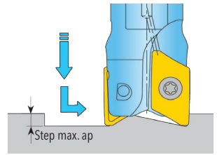
Stechfräsen
